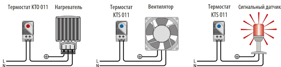
Примеры подключения
